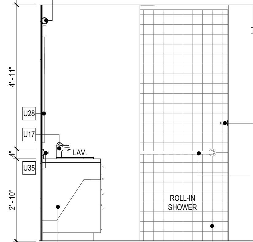
UNIT C-2a ACC. M. BATHROOM ELEV.
