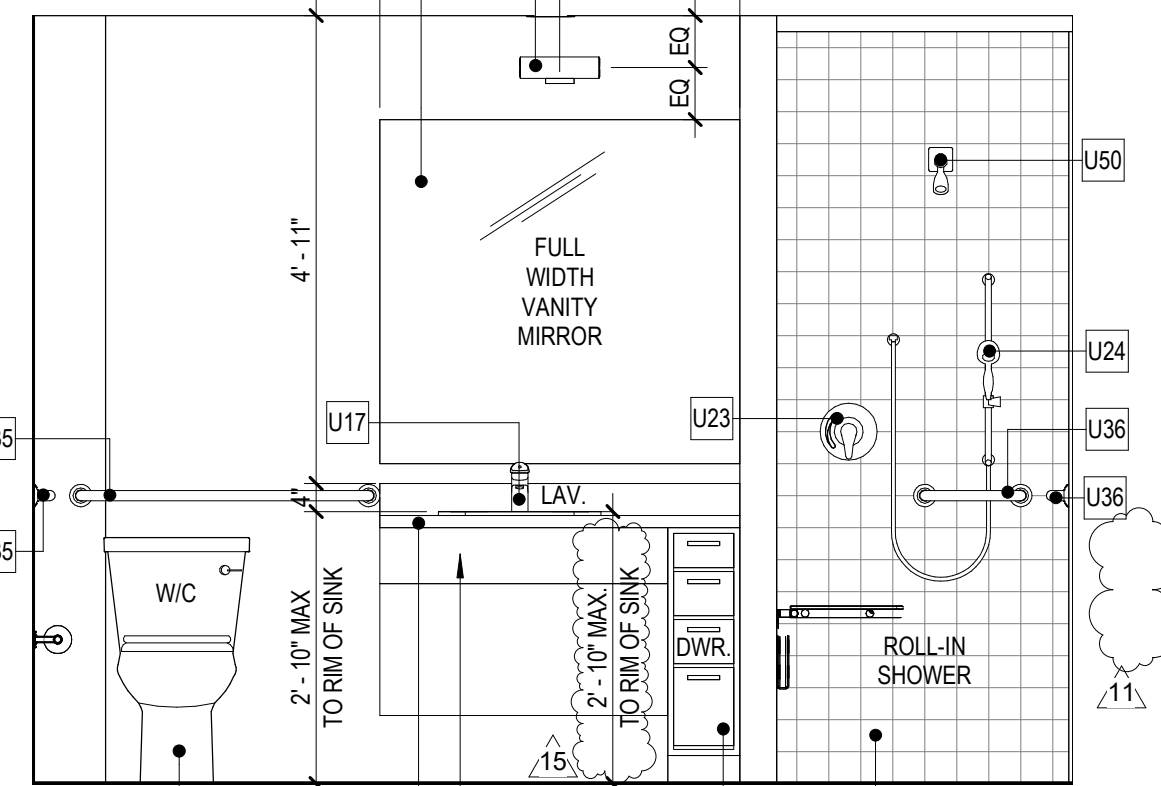
UNIT C-2a ACC. M. BATHROOM ELEV.
